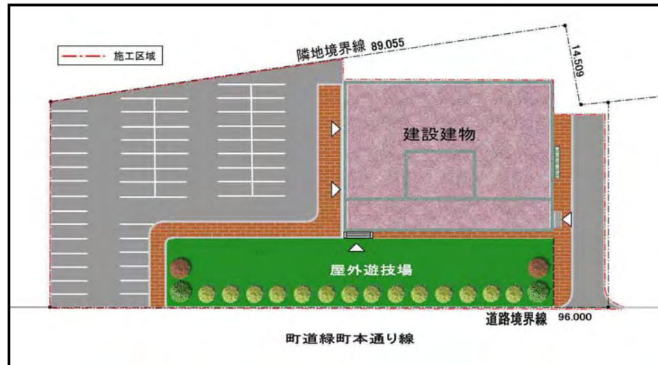
配置図
